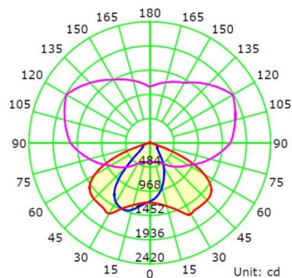
— C0-C180 — C90-C270 — G38 - curbă de distribuție intensitate luminoasă -
